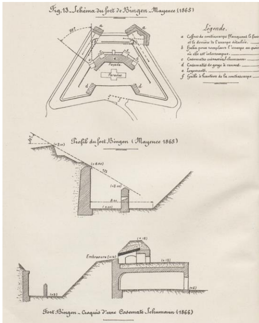
Extrait de la planche V du Cours de Fortification du Lieutenant-Colonel Piarron de Mondésir (La fortification cuirassée et les forteresses du XXème siècle), Paris, décembre 1906
